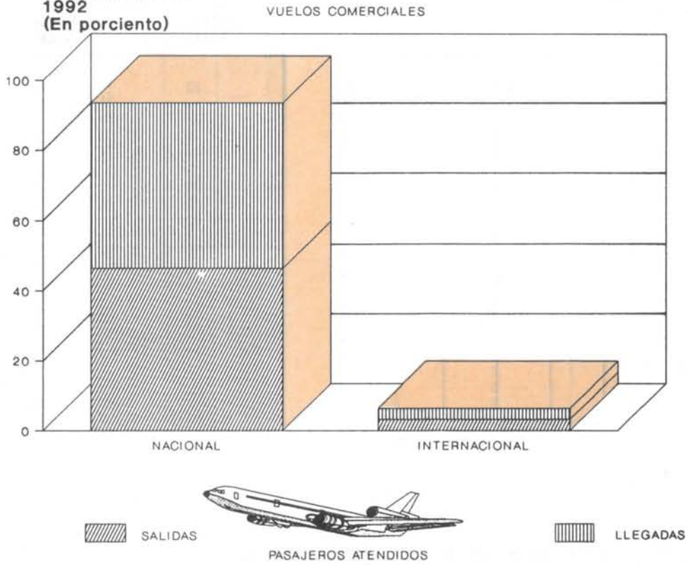
GRAFICA 2.2.5
